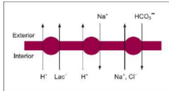
Figura 6-3 Los tres sistemas de transporte de membrana relacionados con la regulación del pH en el músculo esquelético: cotransporte lactato/ H^+ ; intercambio Na^+/H^+ ; sistema de transporte dependiente del CO_3H^- .
