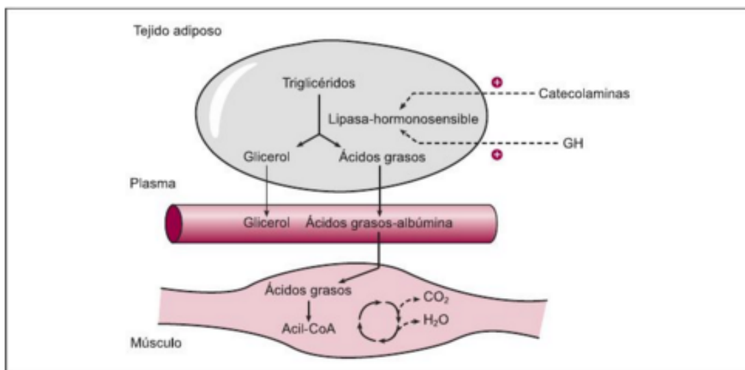
Figura 2-9 Esquema de la activación de la lipólisis iniciada por la acción de la lipasa hormonosensible. GH: hormona del crecimiento.
