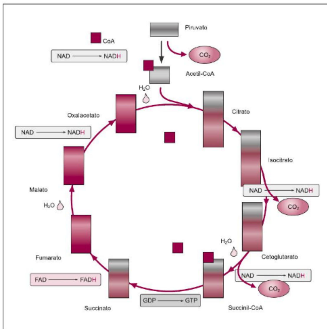
Figura 4-7 Representación esquemática de las reacciones del ciclo de Krebs. El acetil-CoA se incorpora al ciclo uniéndose al oxalacetato para convertirse en citrato. El ciclo consume agua y libera H (reduciendo FAD y NAD) y \text{CO}_2 . FAD: dinucleótido de adenina y flavina. NAD: dinucleótido de adenina nicotinamida. NADH: dinucleótido de adenina nicotinamida reducido. GDP: difosfato de guanosina. GTP: trifosfato de guanosina.
