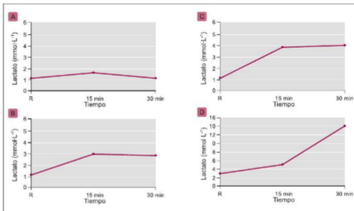
Figura 5-4 Ejemplo de determinación del máximo estado estable del lactato (MLSS). Se muestran las respuestas del lactato en sangre a cuatro distintas velocidades de carrera. A) 14 \text{ km} \cdot \text{h}^{-1} . La concentración de lactato en sangre no se eleva respecto a la de reposo y se muestra estable entre el minuto 15 y 30 de ejercicio. B) 15 \text{ km} \cdot \text{h}^{-1} . La concentración de lactato en sangre se eleva respecto a la de reposo, pero se mantiene estable entre el minuto 15 y 30. C) 16 \text{ km} \cdot \text{h}^{-1} . La concentración de lactato en sangre se eleva respecto a la de reposo, pero se mantiene estable entre el minuto 15 y 30. D) 17 \text{ km} \cdot \text{h}^{-1} . La concentración de lactato en sangre aumenta progresivamente desde el inicio del ejercicio, mostrando que la producción de lactato supera a los procesos de aclaramiento. La intensidad MLSS se sitúa en este ejemplo a 16 \text{ km} \cdot \text{h}^{-1} .
