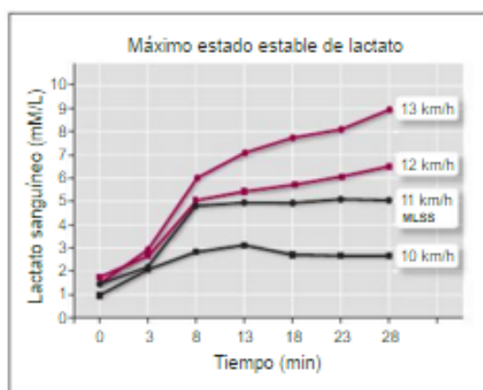
Figura 1-9 Determinación del máximo estado estable del lactato mediante la aplicación de diferentes intensidades durante un tiempo prolongado. La máxima carga asociada a un aumento de los niveles de lactato en sangre inferior a 1 mM/L define el máximo estado estable del lactato (MLSS).
